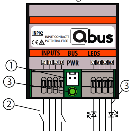
Figuur 2 : Aansluitvoorbeeld van de bus en ingangen
