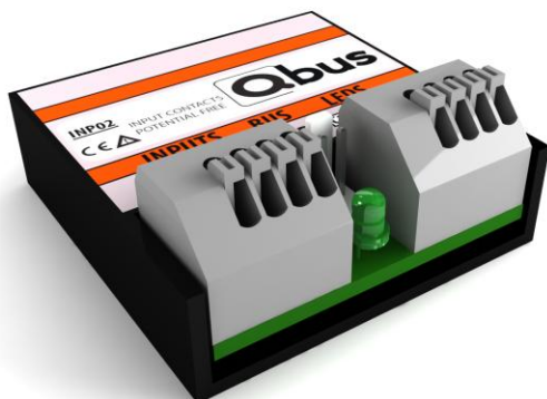
Figuur 1 : Ingangsmodule INP02
