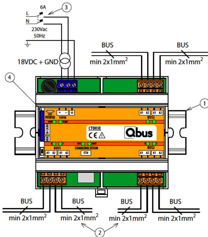
Afbeelding 2: Aansluitingscontroller CTD03E
