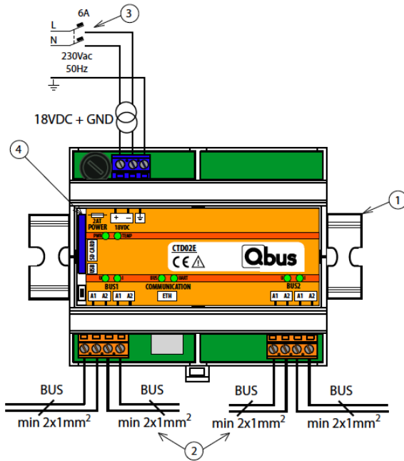
Afbeelding 2: Aansluitingscontroller CTD02E
