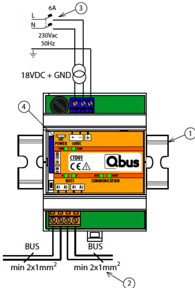
Afbeelding 2: Aansluitingscontroller CTD01
