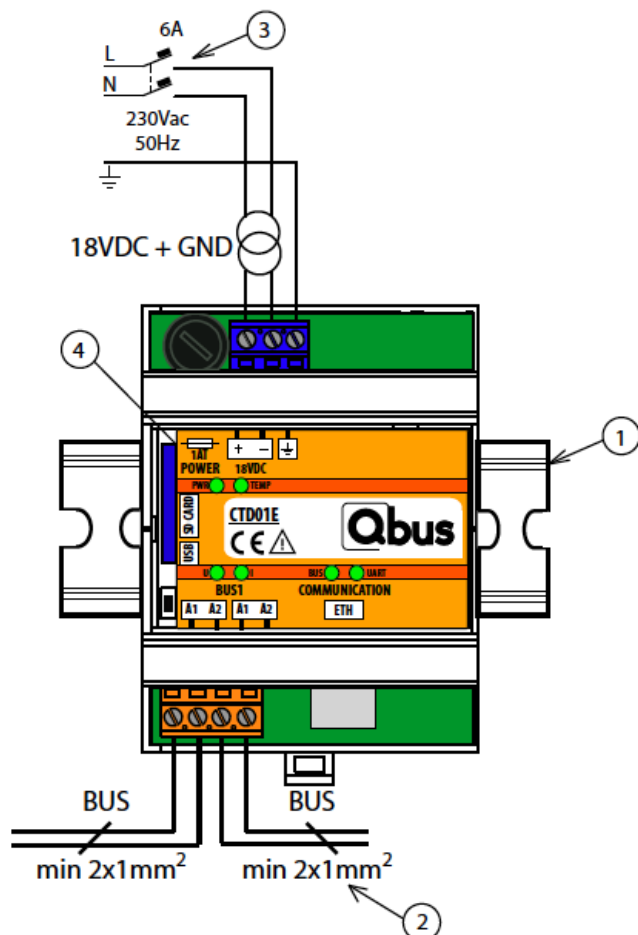
Afbeelding 2: Aansluitingscontroller CTD01E
