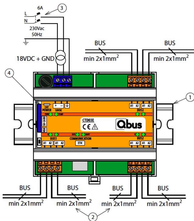
Figure 2 : connection du contrôleur CTD03E
