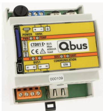
Figure 1 : contrôleur CTD01E+
