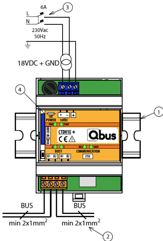
Figure 2 : connection du contrôleur CTD01E+
