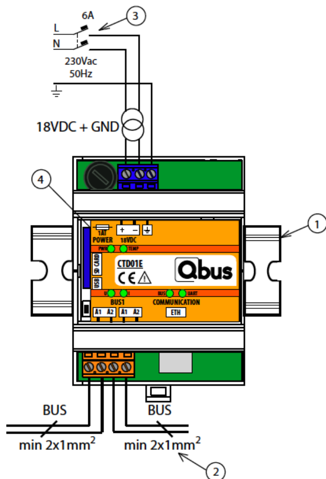
Figure 2 : connexion du contrôleur CTD01E
