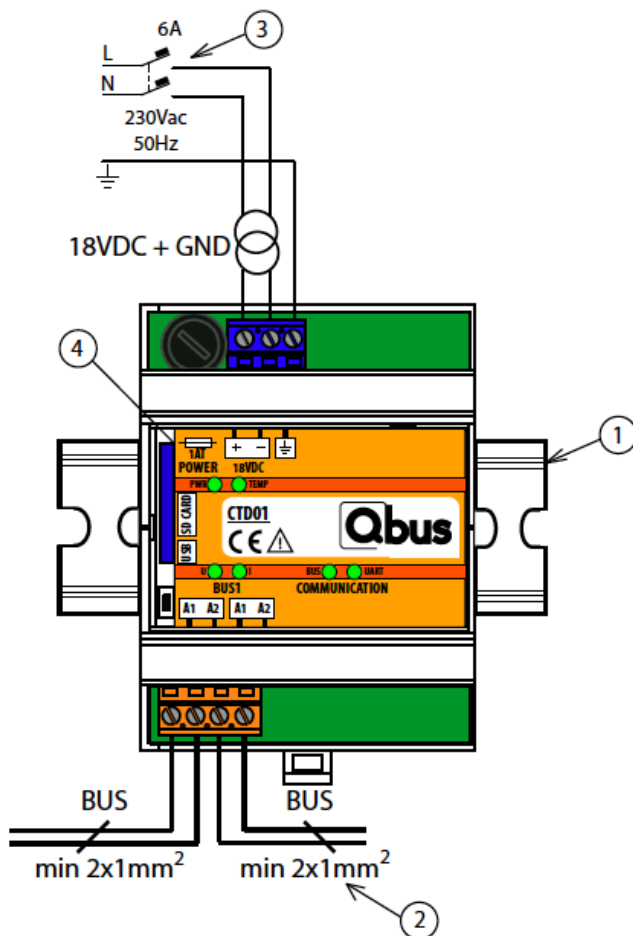
Figure 2 : connection du contrôleur CTD01
