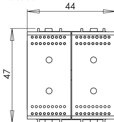
Figure 3 Dimensions interrupteur Bticino® SWC04
