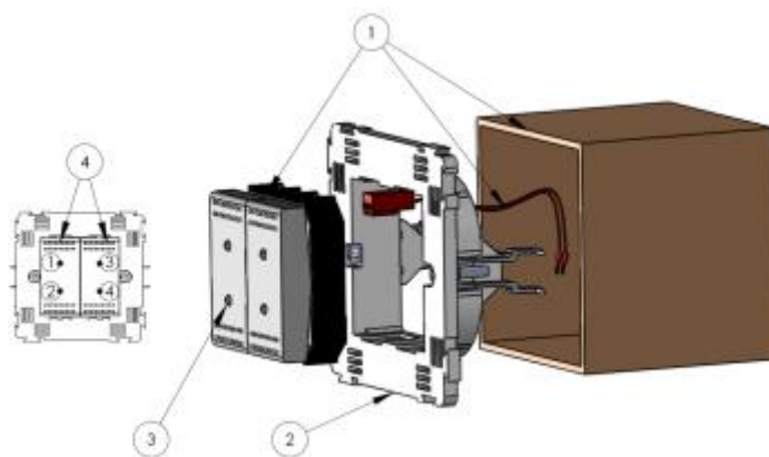
Figure 2 Raccordement de l'interrupteur Bticino® SWC04
