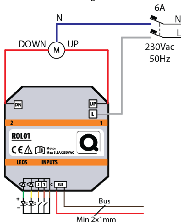
Figure 2 : exemple de raccordement de l'alimentation et des charges
